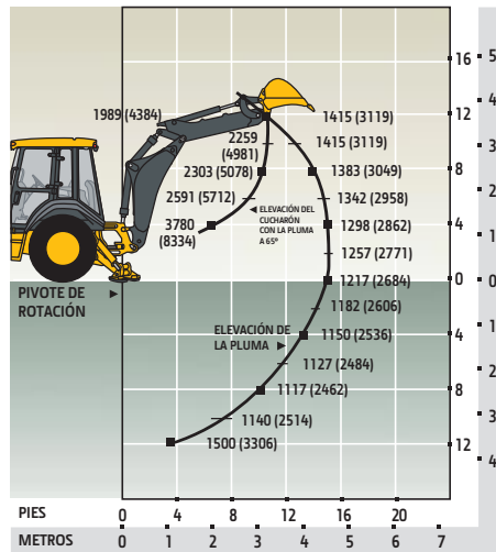
Retroexcavadora 310SK con Brazo de Cucharón Telescópico de 1,07 m (3 ft 6 in) Retraído
