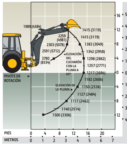
Retroexcavadora 315SK con Brazo de Cucharón Telescópico de 1,07 m (3 ft 6 in) Retraído
