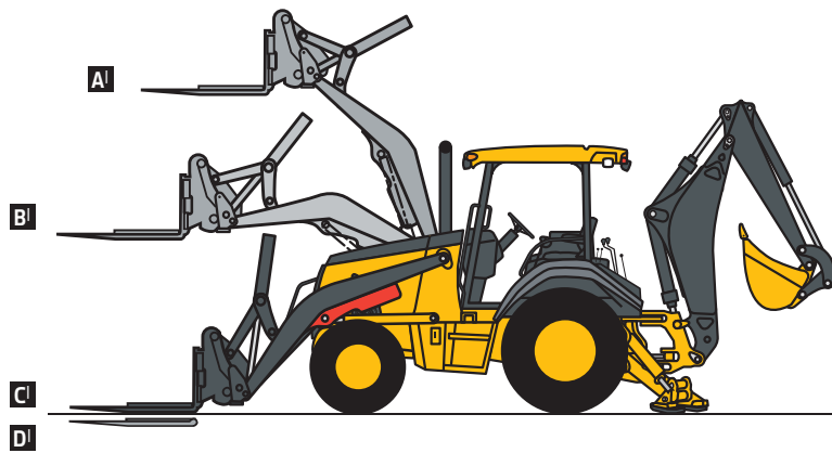
Retroexcavadora 310K con Brazo de Cucharón Telescópico de 1,07 m (3 ft 6 in) Retraído
