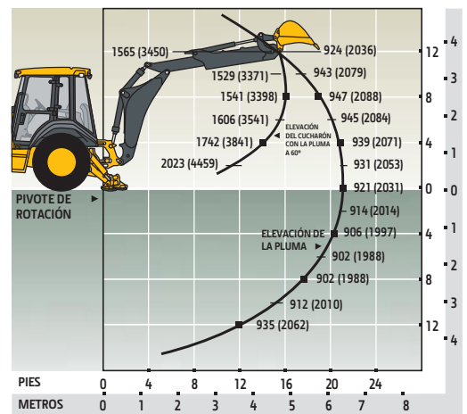
Retroexcavadora 410K con Brazo de Cucharón Telescópico de 1,22 m (4 ft) Extendido
