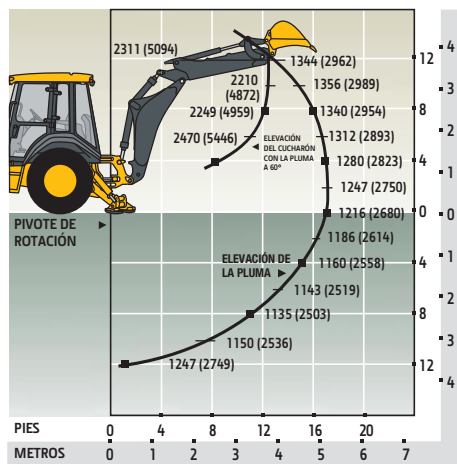
Retroexcavadora 410K con Brazo de Cucharón Telescópico de 1,22 m (4 ft) Retraído
