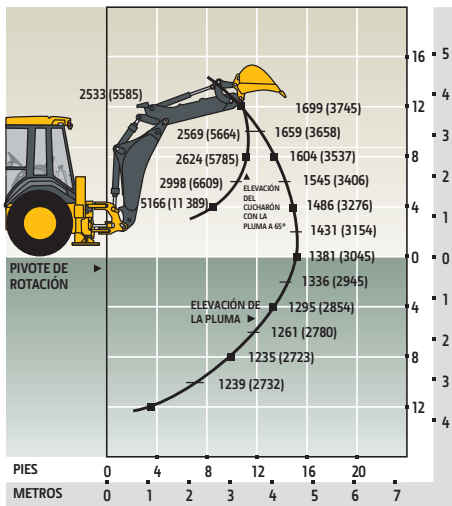
Retroexcavadora 315SK con Brazo de Cucharón Estándar
