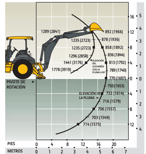
Retroexcavadora 310K con Brazo de Cucharón Telescópico de 1,07 m (3 ft 6 in) Extendido
