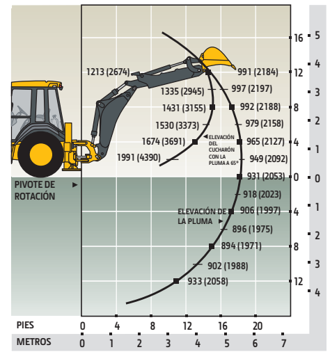
Retroexcavadora 315SK con Brazo de Cucharón Telescópico de 1,07 m (3 ft 6 in) Extendido
