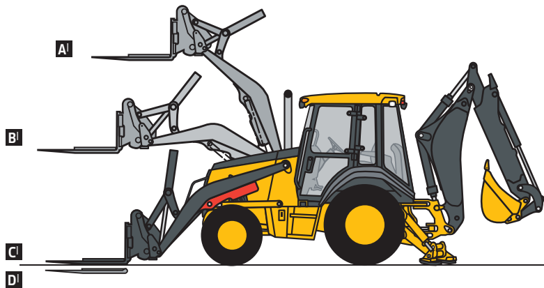
Retroexcavadora 310SK con Brazo de Cucharón Telescópico de 1,07 m (3 ft 6 in) Retraído
