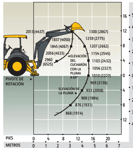
Retroexcavadora 310K con Brazo de Cucharón Telescópico de 1,07 m (3 ft 6 in) Retraído
