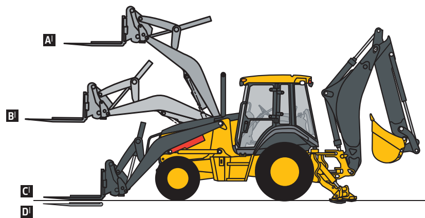
Retroexcavadora 710K con Brazo de Cucharón Telescópico de 1,37 m (4 ft 6 in) Retraído
