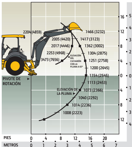
Retroexcavadora 310K con Brazo de Cucharón Estándar
