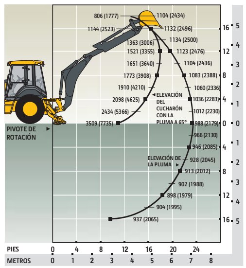
Retroexcavadora 710K con Brazo de Cucharón Telescópico de 1,37 m (4 ft 6 in) Extendido
