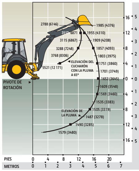
Retroexcavadora 710K con Brazo de Cucharón Estándar
