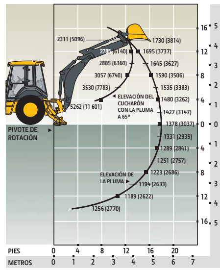
Retroexcavadora 710K con Brazo de Cucharón Telescópico de 1,37 m (4 ft 6 in) Retraído
