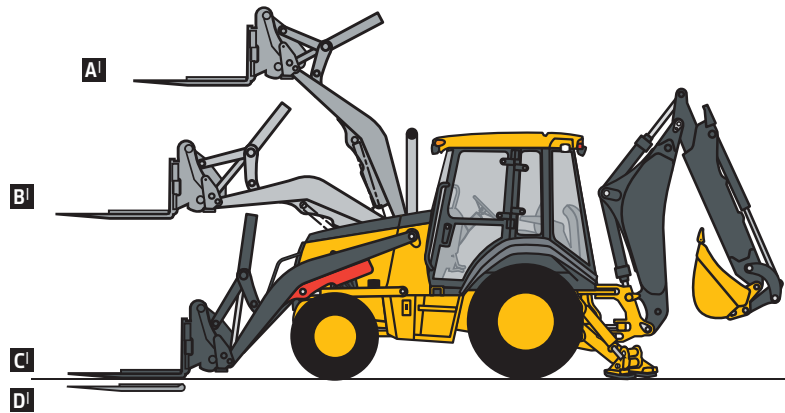
Retroexcavadora 410K con Brazo de Cucharón Telescópico de 1,22 m (4 ft) Retraído
