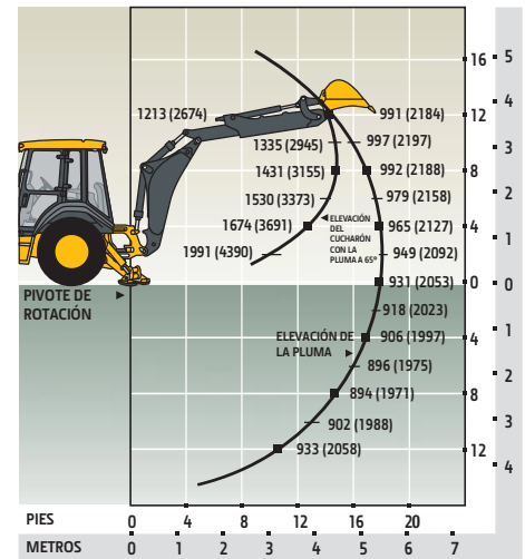
Retroexcavadora 310SK con Brazo de Cucharón Telescópico de 1,07 m (3 ft 6 in) Extendido
