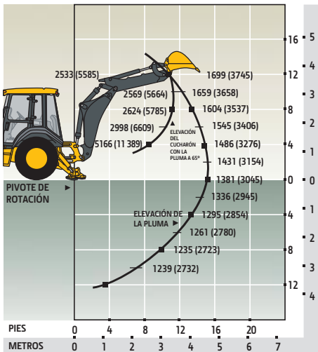
Retroexcavadora 310SK con Brazo de Cucharón Estándar
