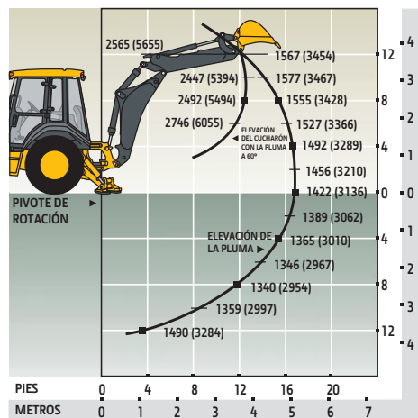
Retroexcavadora 410K con Brazo de Cucharón Estándar
